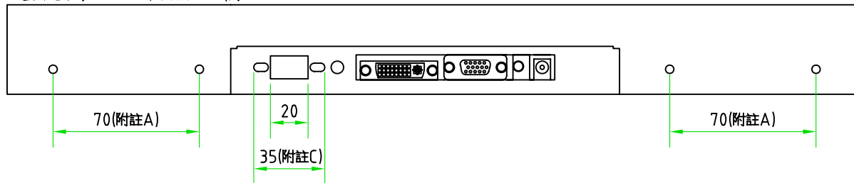
底視圖 -- 液晶面朝上
