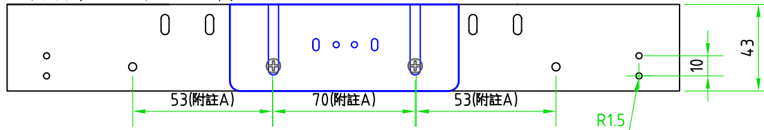
側視圖 -- 液晶面朝上
